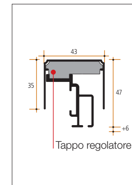
Compensatore a guida montata.
