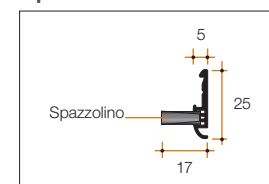
Profilo di riscontro.
